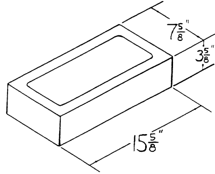
8×4×16 WEBLESS
