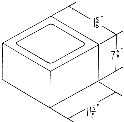
12×8×12 WEBLESS
