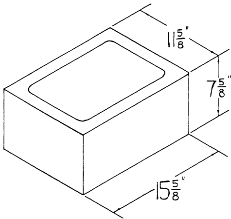
12×8×16 WEBLESS
