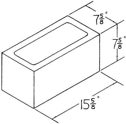
8×8×16 WEBLESS
