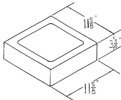
12×4×12 WEBLESS
