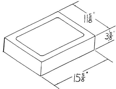
12×4×16 WEBLESS
